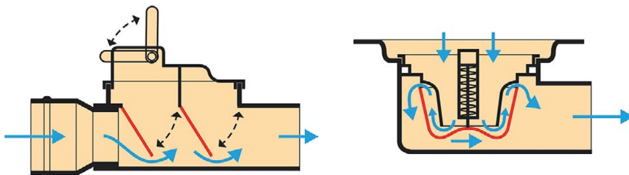
Illustrationen till vänster visar en backventil med en eller två ventilkaffar. Den till höger är en skiss av en självstängande golvbrunn.
